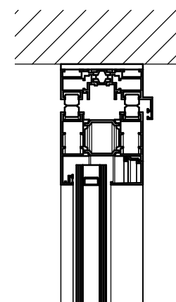
6 Detail 4 1 : 5
