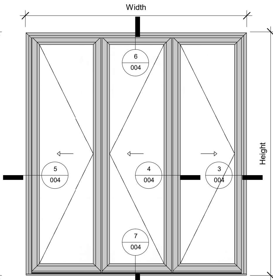
2 Elevation Back 1 : 20
