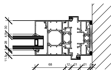
5 Detail 3 1 : 5
