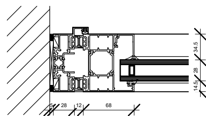
3 Detail 1 1 : 5
