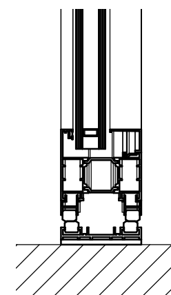
7 Detail 5 1 : 5
