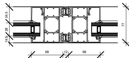
4 Detail 2 1 : 5
